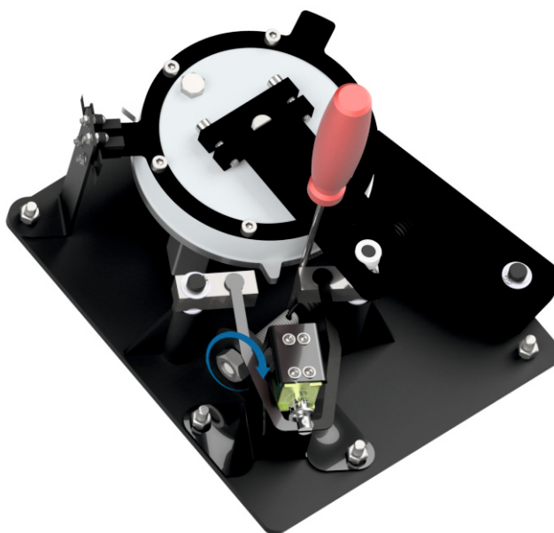
Рисунок 12.4.1 – Регулировка натяжения пружины доводчика
